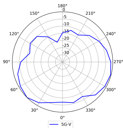
5GHz (垂直)
