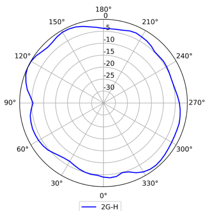
2.4GHz (水平)
