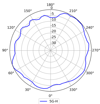
5GHz (水平)
