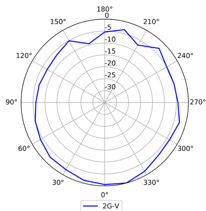
2.4GHz (垂直)
